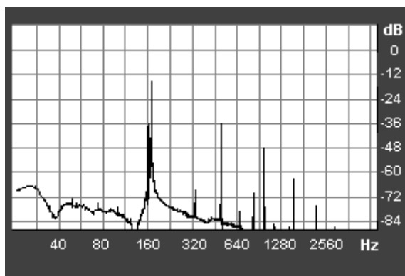
Rys. 4. Widmo dźwięku misy nr 2
