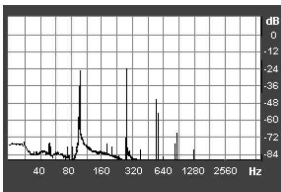
Rys. 6. Widmo dźwięku misy nr 3
