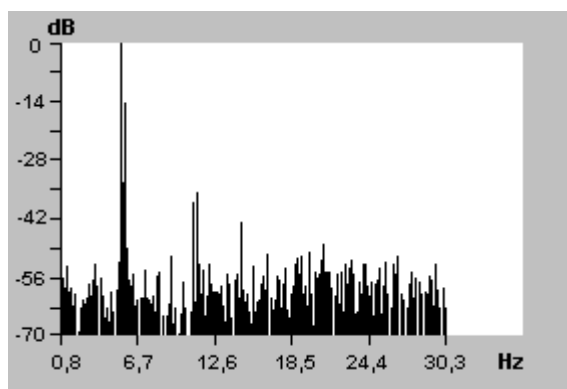
Rys. 3. Widmo obwiedni dźwięku misy nr 1
