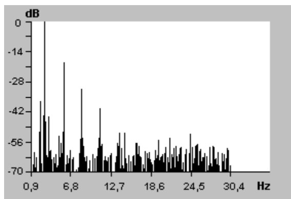
Rys. 7. Widmo obwiedni dźwięku misy nr 3
